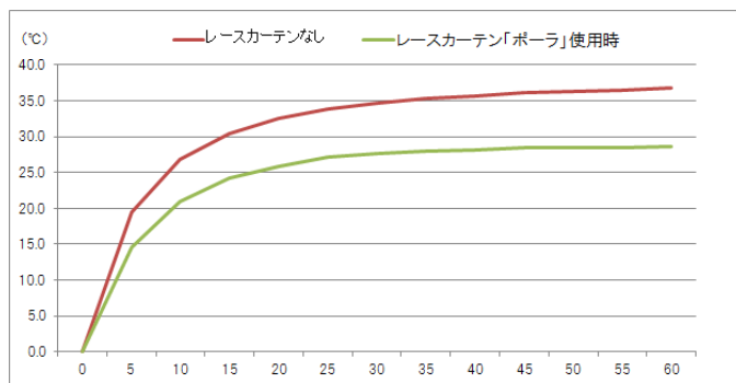
左:レースカーテン「ポーラ」製品使用イメージ 右:赤外ランプ 60℃法による室温上昇推移グラフ
